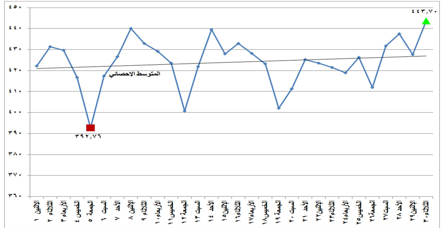
شكل (١٧) الطاقة الكهربائية المنتجة من الغاز الطبيعي خلال شهر ابريل ٢٠١٩
