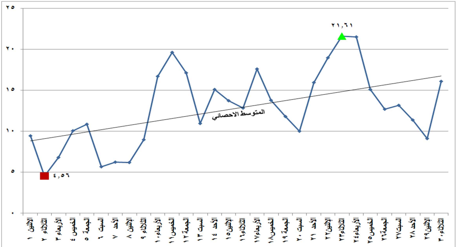
شكل (٢٥) الطاقة الكهربائية المنتجة من الرياح والشمس خلال شهر ابريل ٢٠١٩
