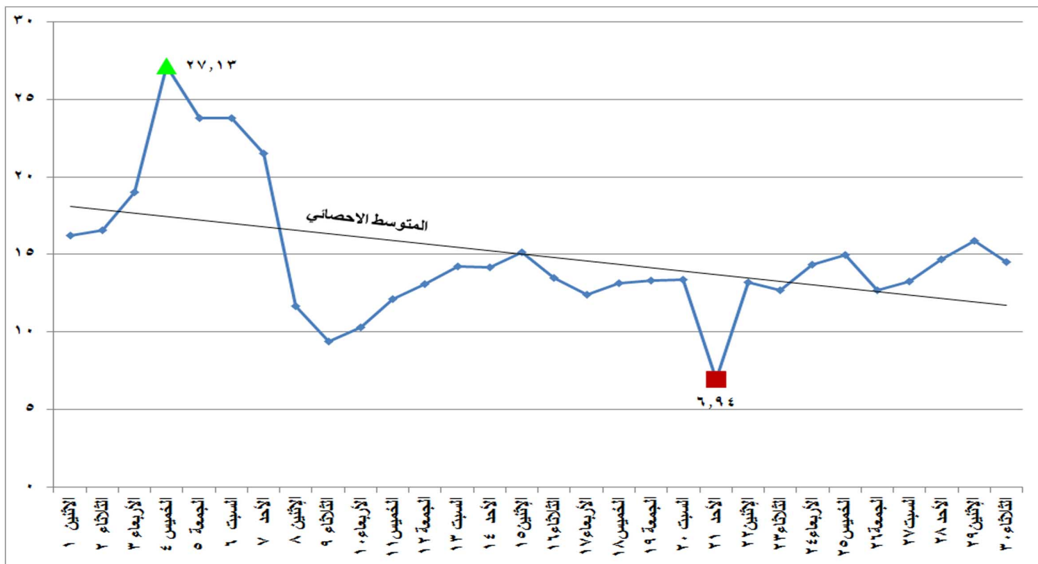
شكل (١٩) الطاقة الكهربائية المنتجة من المازوت خلال شهر ابريل ٢٠١٩
