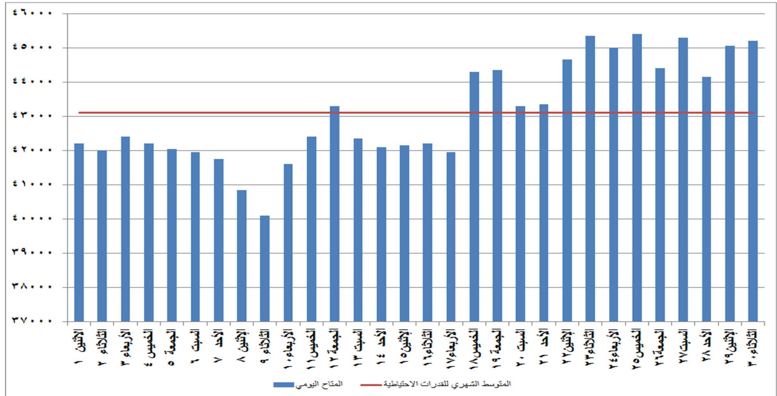
شكل (٢٧) القدرات المتاحة يوميا والمتوسط الشهري للقدرة الاحتياطية خلال شهر ابريل ٢٠١٩
