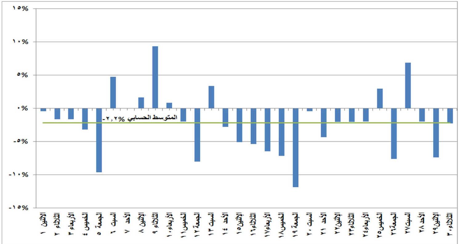
شكل (٩) النسب المئوية للتغير في الحمل الاقصى خلال شهر ابريل ٢٠١٩ مقارنة باليوم المماثل من العام الماضي
