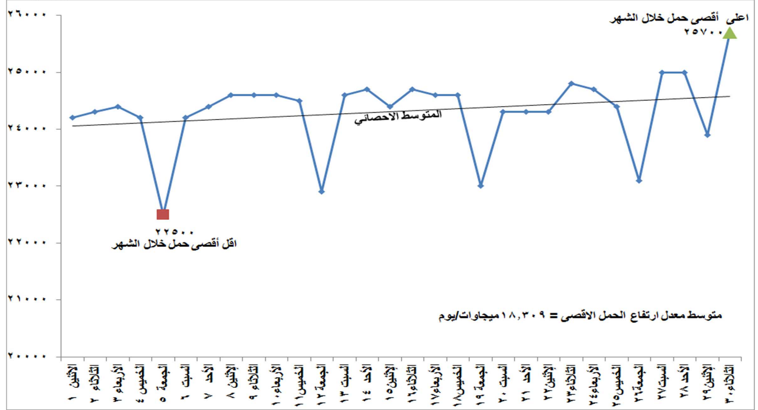
شكل (١) تطور الحمل الاقصى اليومي خلال شهر ابريل ٢٠١٩
