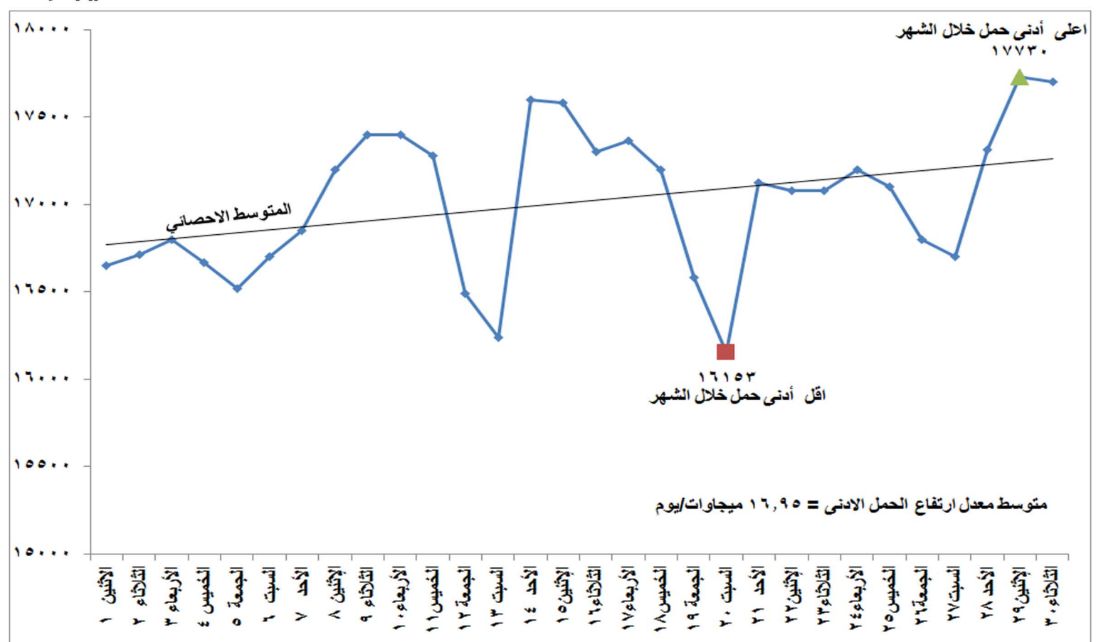
شكل (٢) تطور الحمل الادنى اليومي خلال شهر ابريل ٢٠١٩
