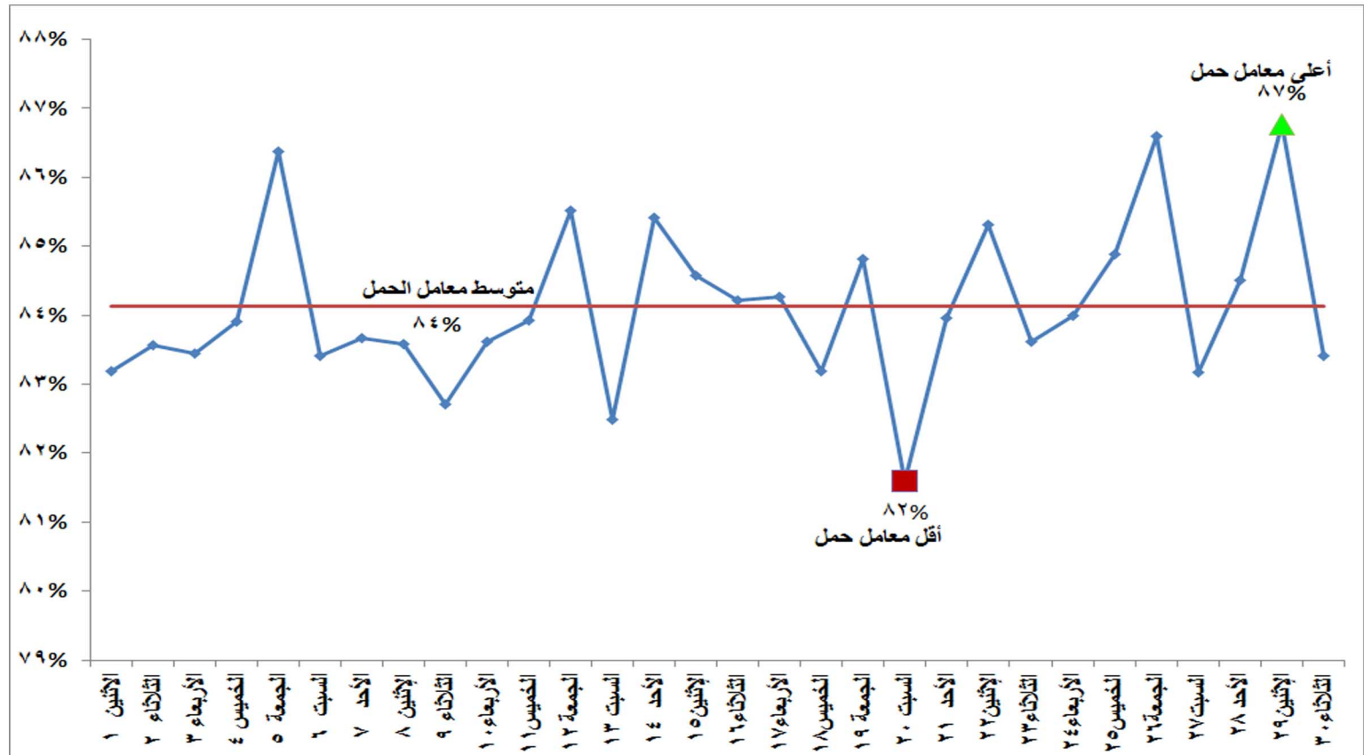
شكل (١٢) إجمالي معامل الحمل لوحدات الانتاج خلال شهر ابريل ٢٠١٩
