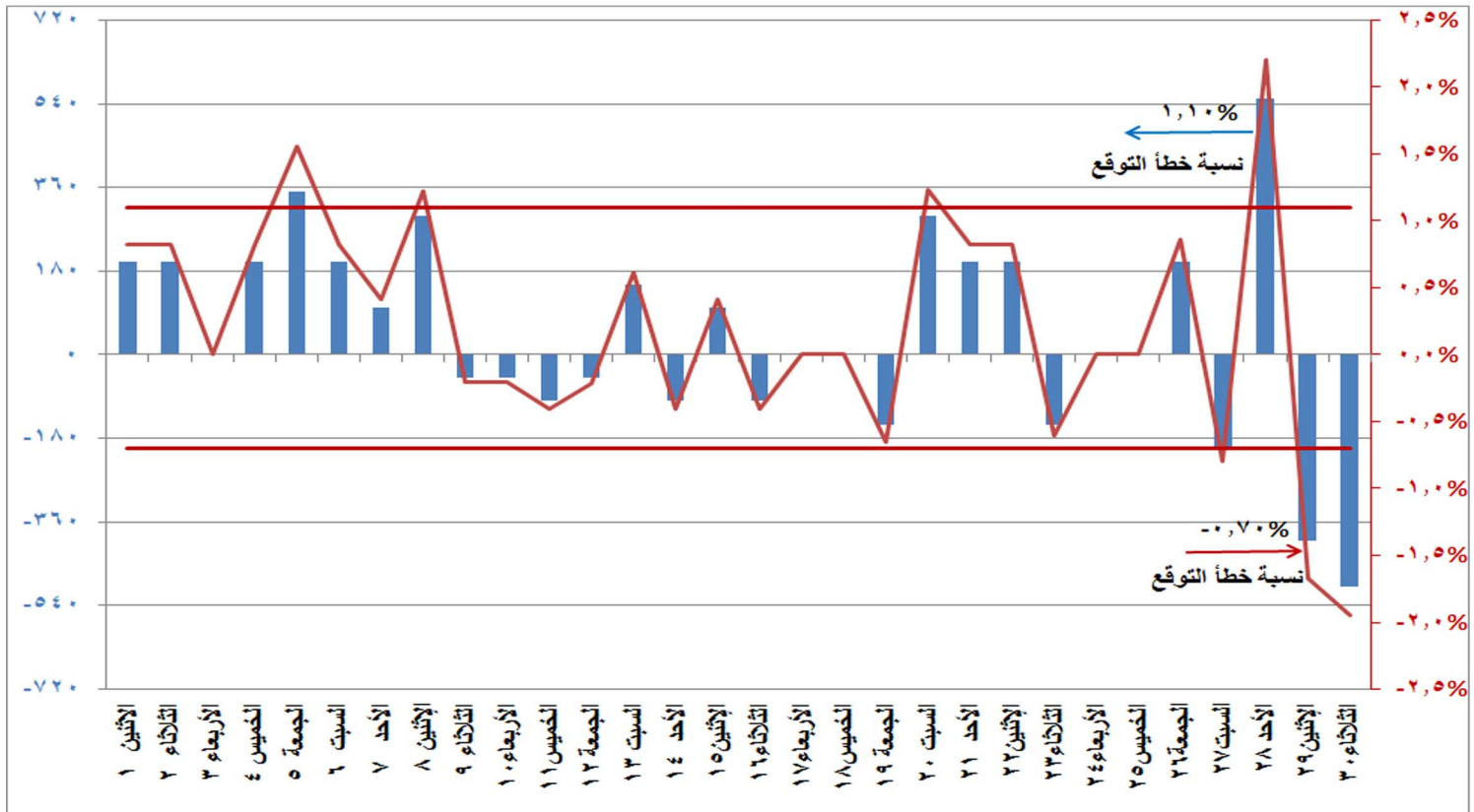
شكل (١٠) الفرق بين الحمل الأقصى المتوقع والمسجل فعليا ونسبة الفرق إلى الحمل المسجل فعليا خلال شهر ابريل ٢٠١٩
