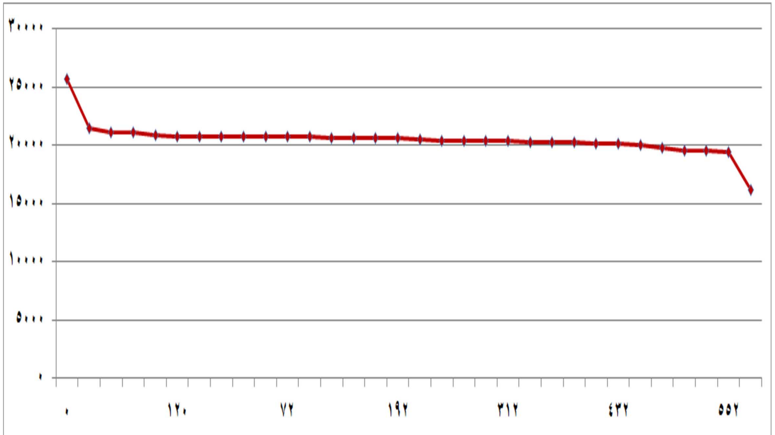
شكل (٨) المنحنى الشهري لفترة الحمل ابريل ٢٠١٩
