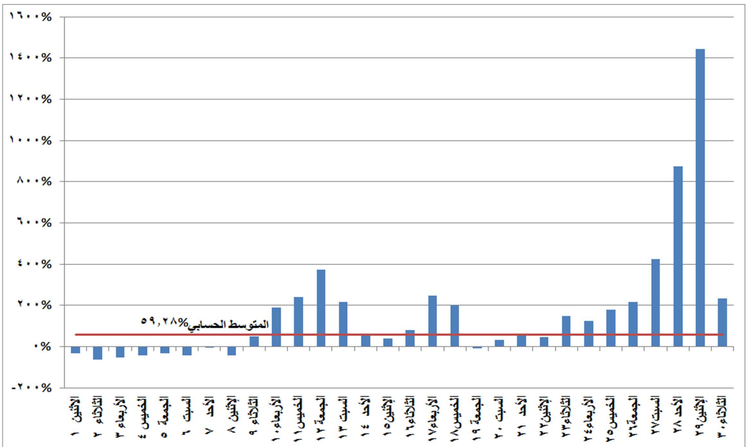
شكل (٢٦) نسب التغير في استخدام الرياح والشمس في إنتاج الطاقة الكهربائية خلال شهر ابريل ٢٠١٩ مقارنة بالشهر المماثل من العام السابق
