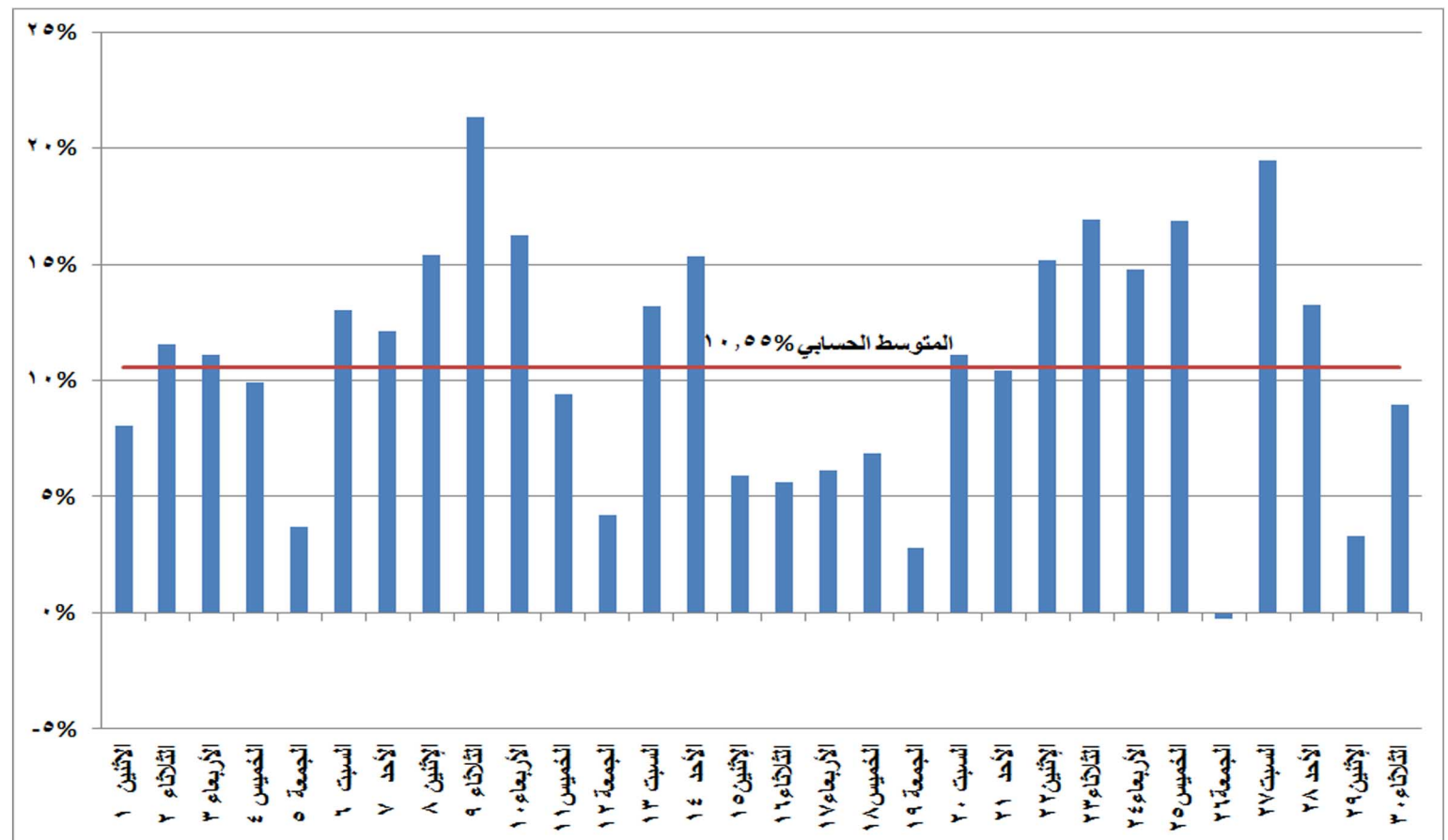
شكل (١٨) نسب التغير في استخدام الغاز الطبيعي في إنتاج الطاقة الكهربائية خلال شهر ابريل ٢٠١٩ مقارنة بالشهر المماثل من العام السابق
