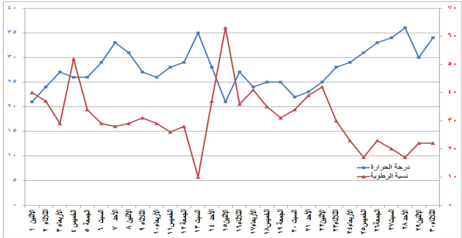
شكل (١١) التغيير في درجة الحرارة والرطوبة النسبية خلال شهر ابريل ٢٠١٩
