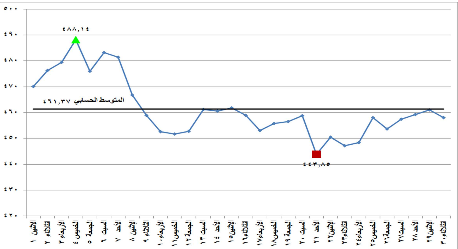
شكل (١٤) معامل انبعاثات غاز ثاني اكسيد الكربون المكافئ على مدى شهر ابريل ٢٠١٩
