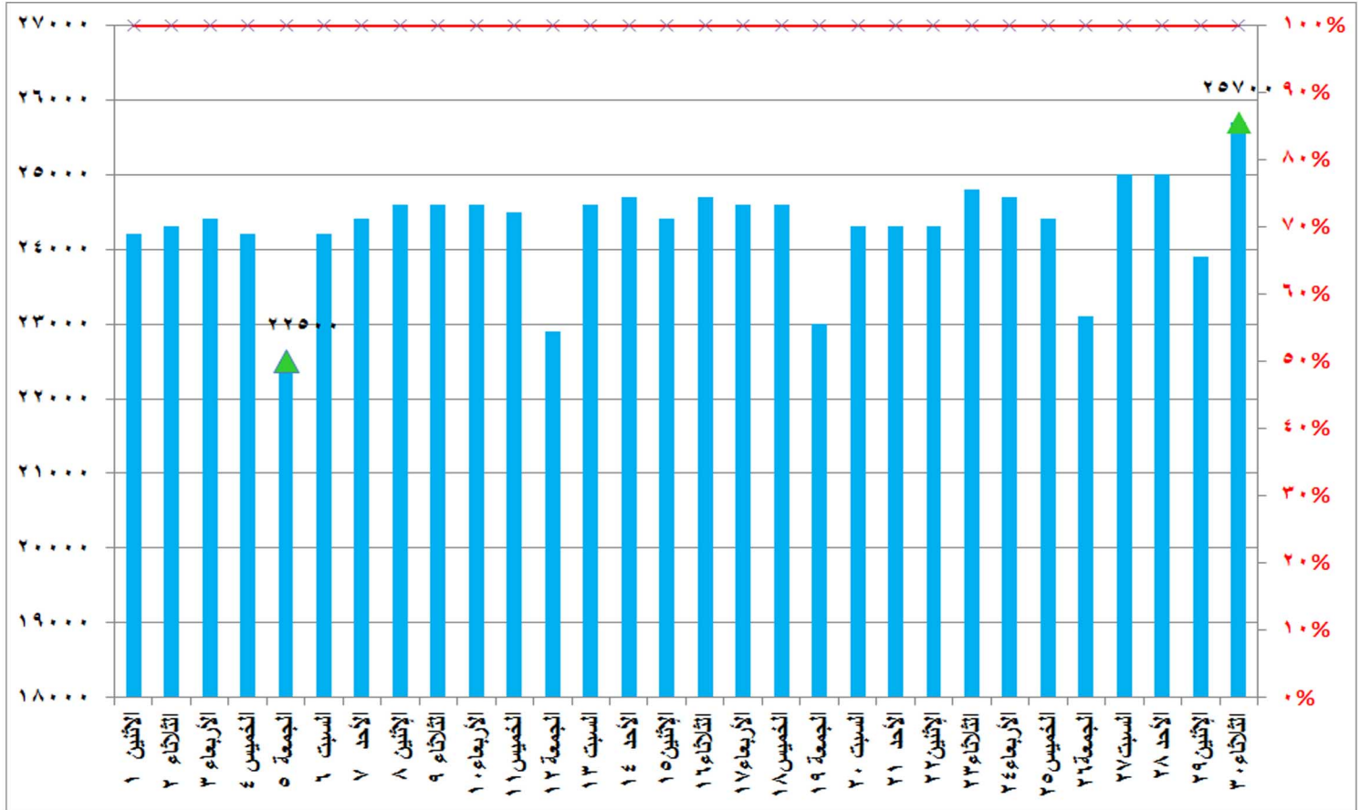
شكل (٥) قدرات الانتاج المتاحة ونسبتها للحمل الأقصى خلال شهر ابريل ٢٠١٩
