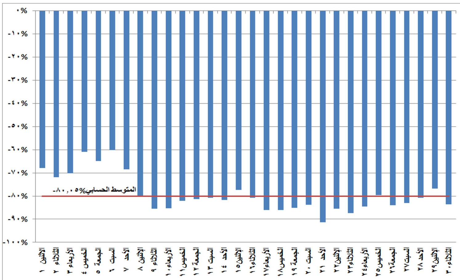
شكل (٢٠) نسب التغير في استخدام المازوت في إنتاج الطاقة الكهربائية خلال شهر ابريل ٢٠١٩ مقارنة بالشهر المماثل من العام السابق
