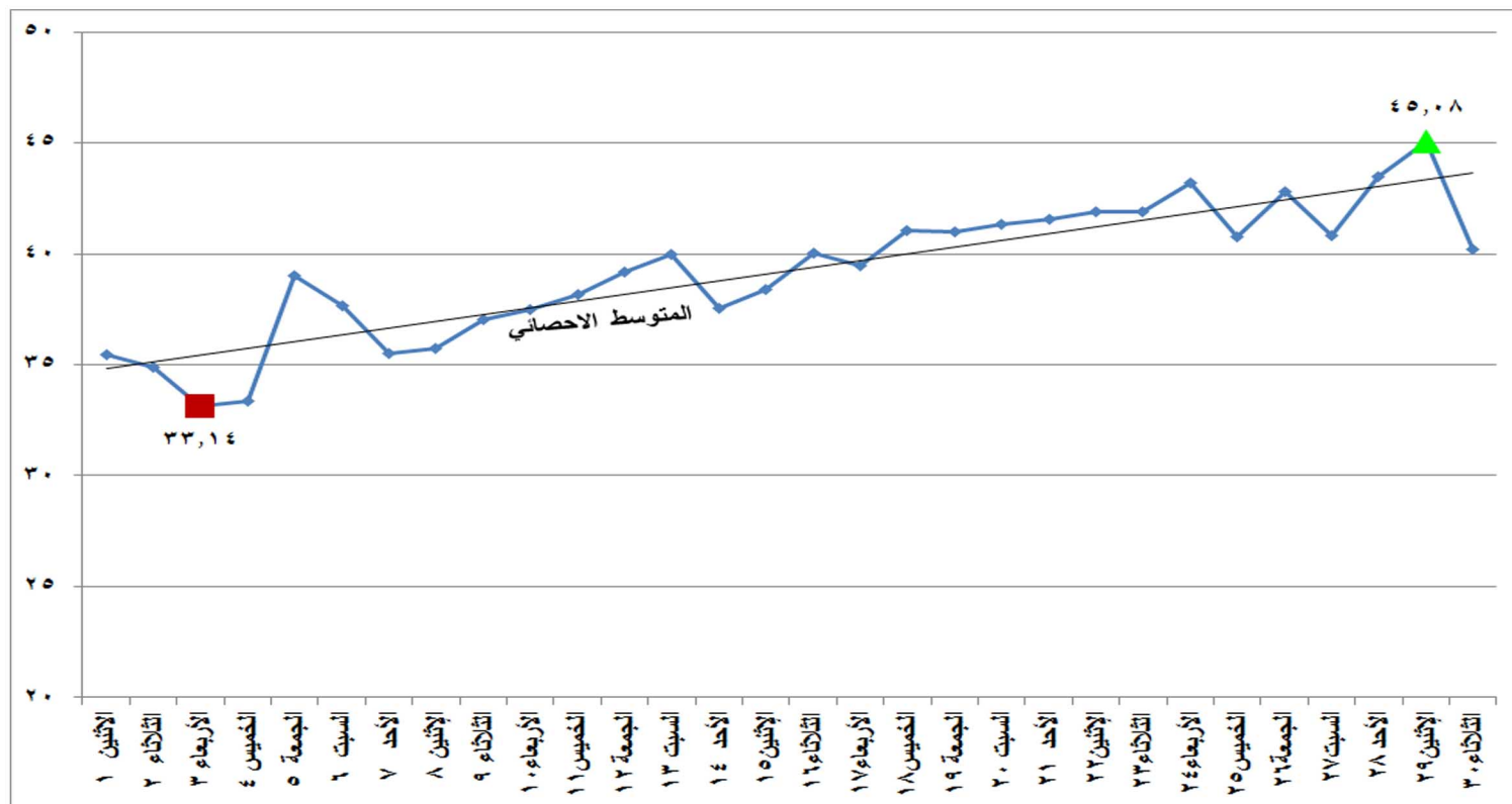
شكل (٢٣) الطاقة الكهربائية المنتجة من المصادر المائية خلال شهر ابريل ٢٠١٩
